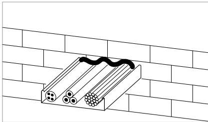
Bild 5, Variante 1: Wulst
