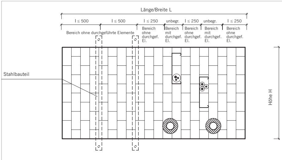
Bild 5: (Schottdicke 200 mm)
